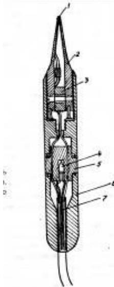
Бесконтактный магнеторезистивный зонд детектора коротких замыканий 1. Магнеторезистор. 2. Магнетодиод. 3. Постоянный магнит. 4. Индикаторная лампочка. 5. Индикаторное окошко. 6. Держатель. 7. Соединительные проводки.
